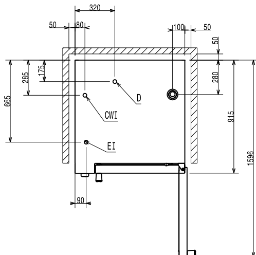
Boven aanzicht
